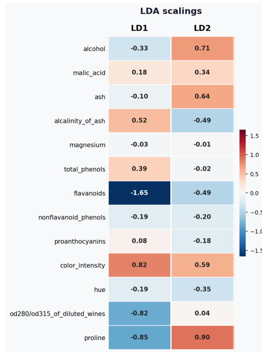
Слика 6: Топлотна мапа доприноса сваке карактеристике дискриминантима LD1 и LD2 код LDA.
